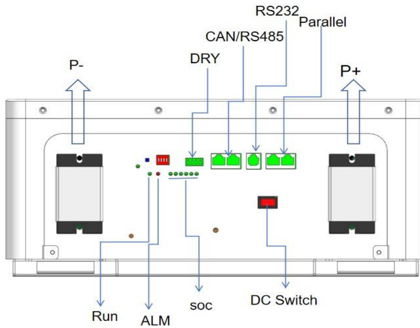
并联通讯端口
